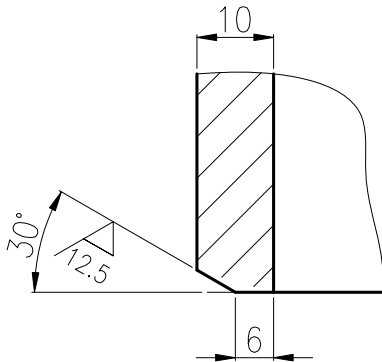
Detail I (详图 I)
